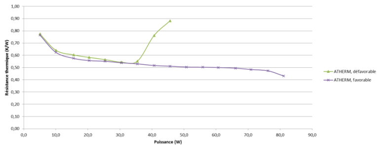
Performances caloduc \varnothing 8\text{ mm} en U ATHERM
